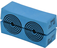
Roxtec-Module GM mit Multidiameter™
